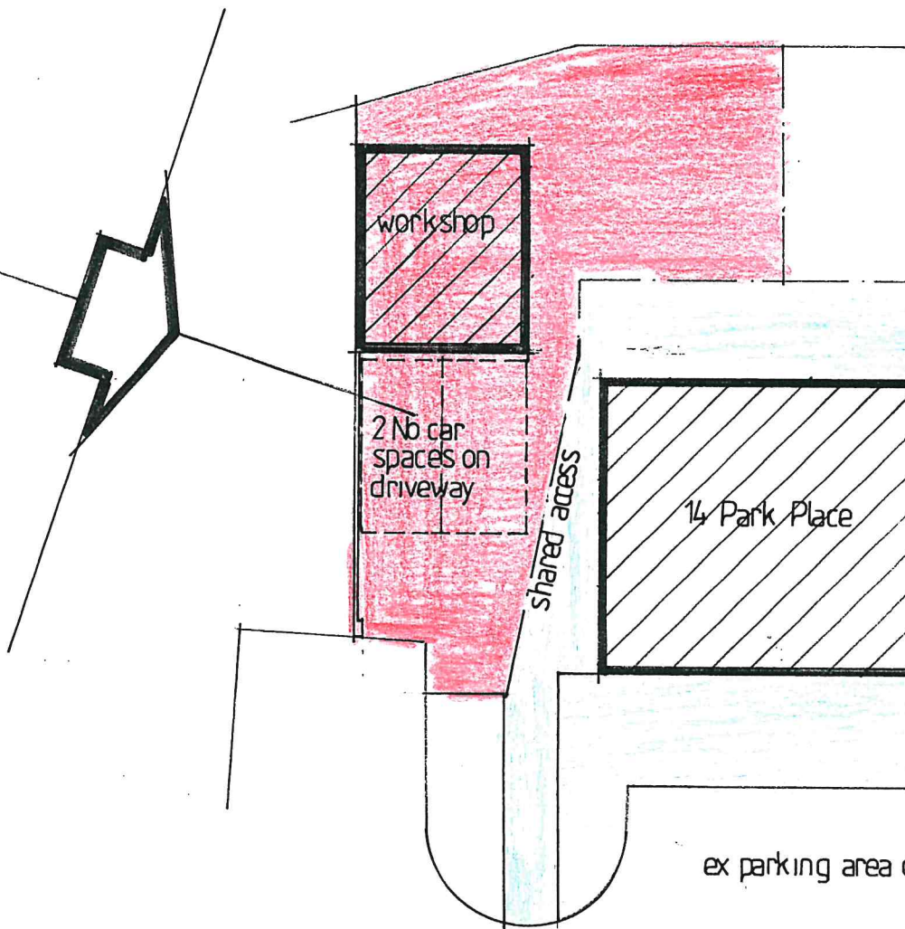
Site plan 1:200
